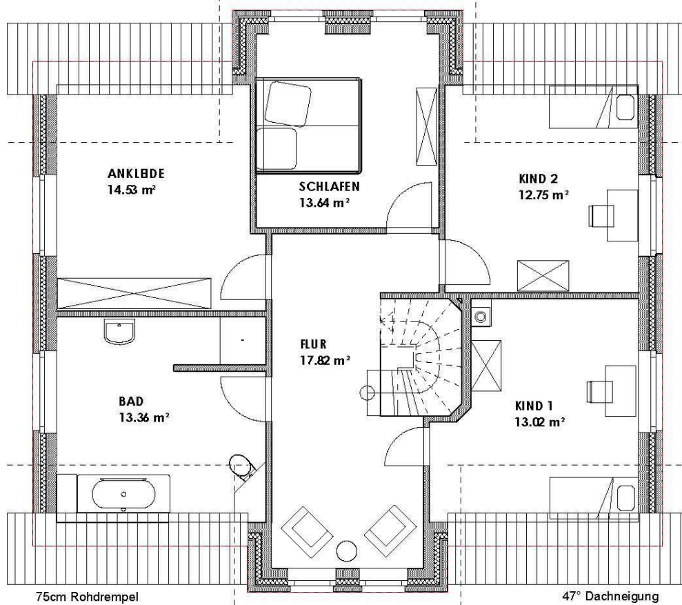
Dachgeschossfläche 85,12 m 2
