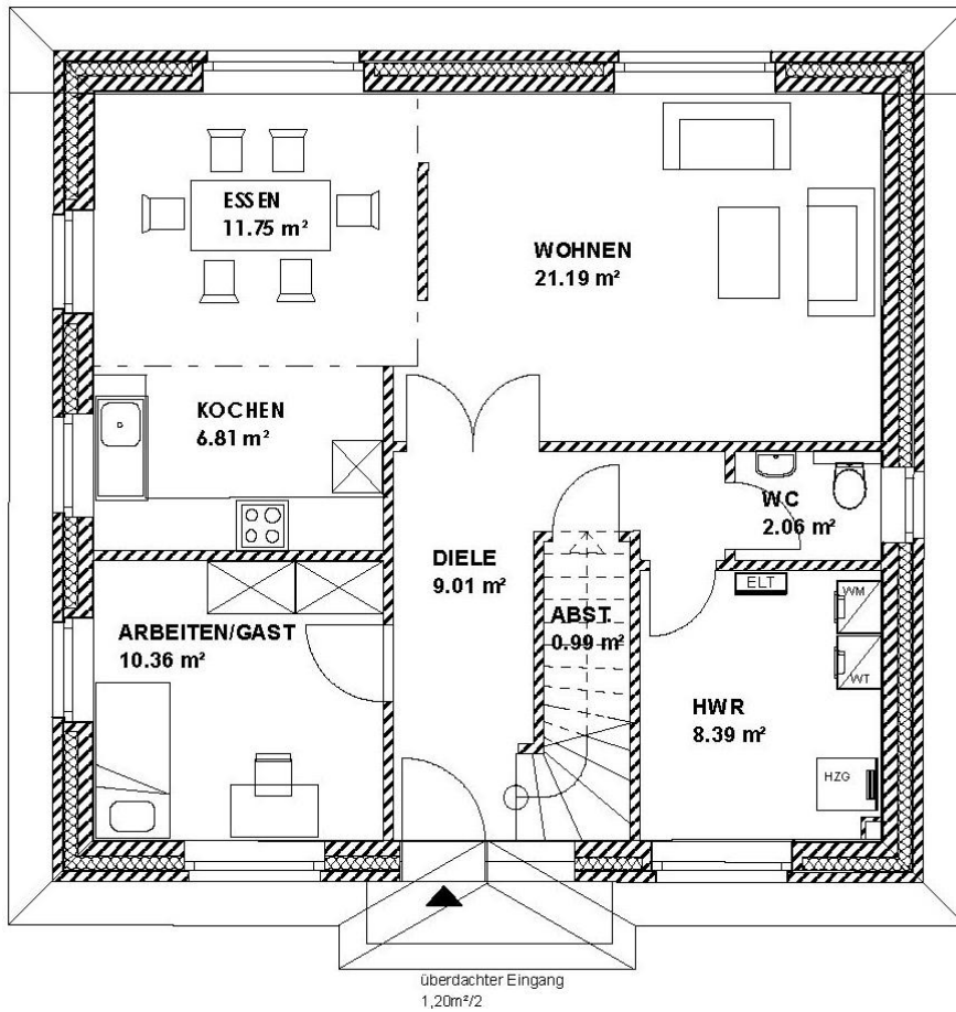
Erdgeschoss Wfl. ca 71,16 m²
