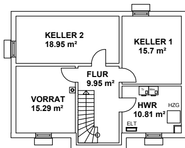
KELLERGESCHOSS Variante (70,70 m 2 WoFl)
