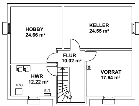
KELLERGESCHOSS Variante (89,09 m 2 WoFI)
