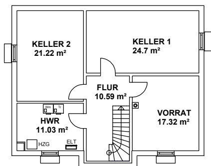
KELLERGEOSCHOSS Variante (84,86 m 2 WoFI)
